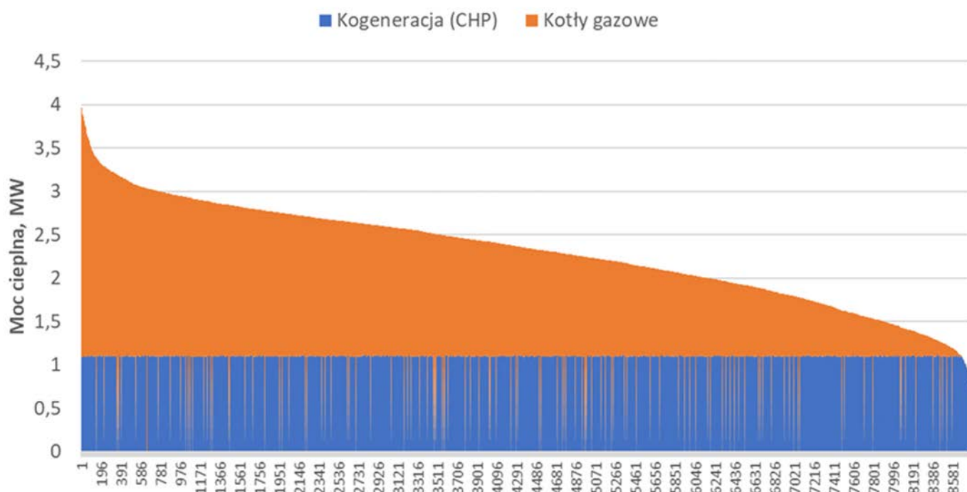
Rysunek 5. Uporządkowany wykres godzinowy pokrycia zapotrzebowania na moc cieplną w zakładzie produkcji wyrobów czekoladowych przed modernizacją
